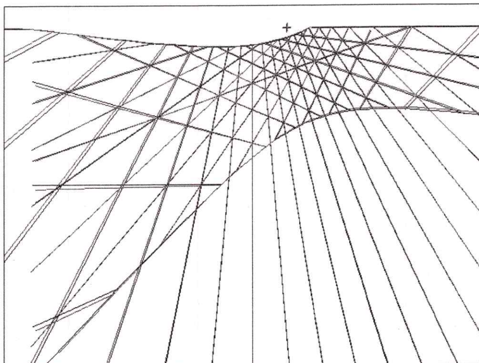
Fig. 6. Het berekende tafereel met de plaatselijke tijd per half uur, Babylonische en Italiaanse tijd per uur, en de drie primaire datumlijnen, voor declinaties van 27^{\circ}20' (de ontwerptekening, blauw) en 27^{\circ}49' (de zonnewijzer, rood, er bovenop). De 12-uurs lijnen zijn op elkaar gelegd op het snijpunt met de equinoxlijn. De plusjes zijn de voetpunten van de gnomons.
