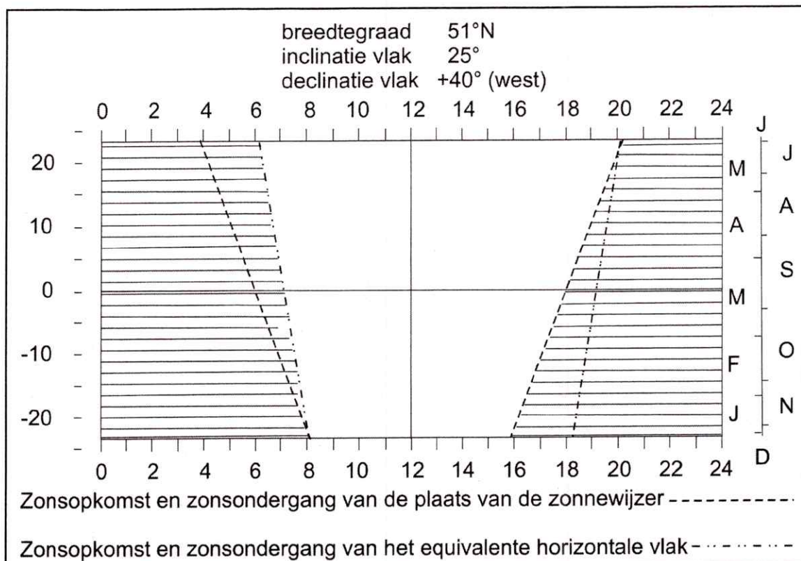
Figuur 5: de uiterste uren van zonnenschijn voor het vlak in ons voorbeeld bij de herleiding.
